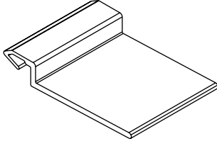
Jamb Extension Clip Extrusion #1076-V
